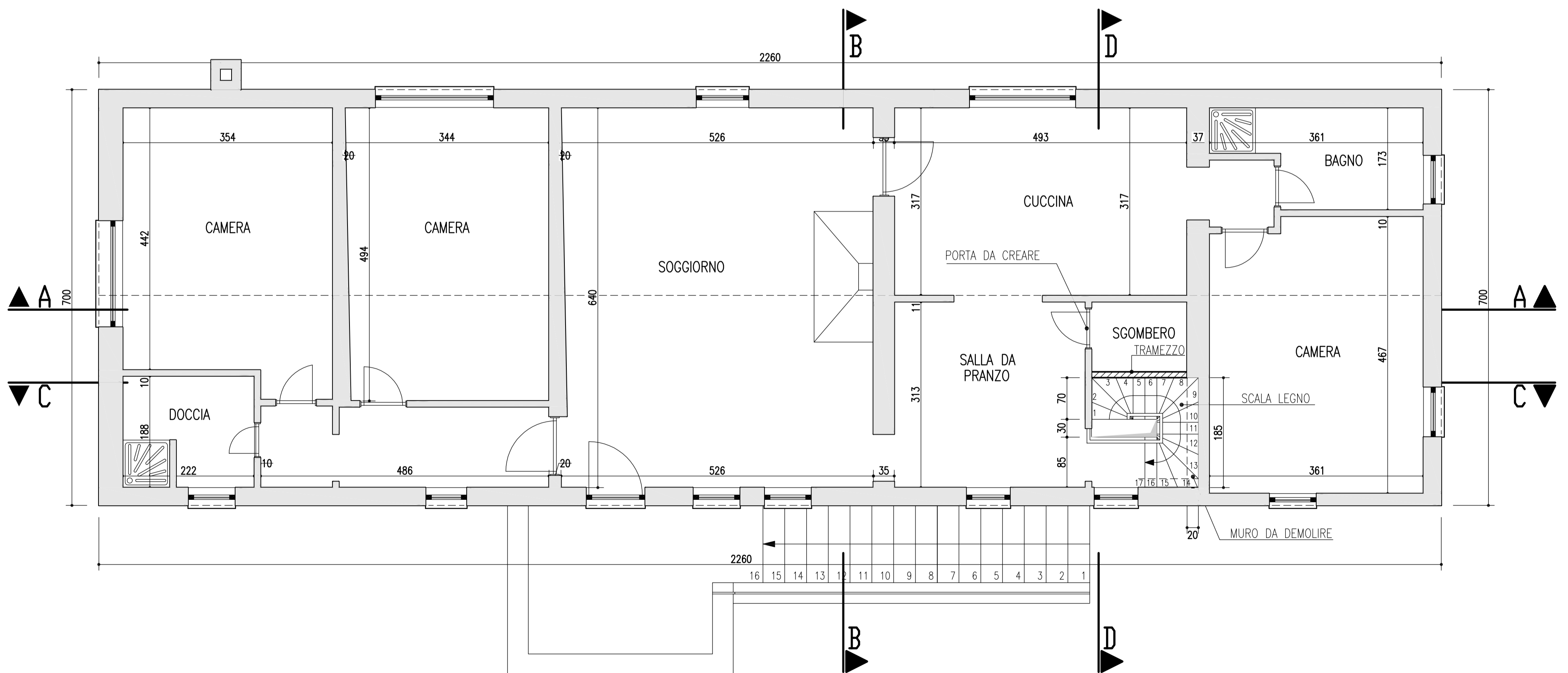
PIANO RIALZATO
